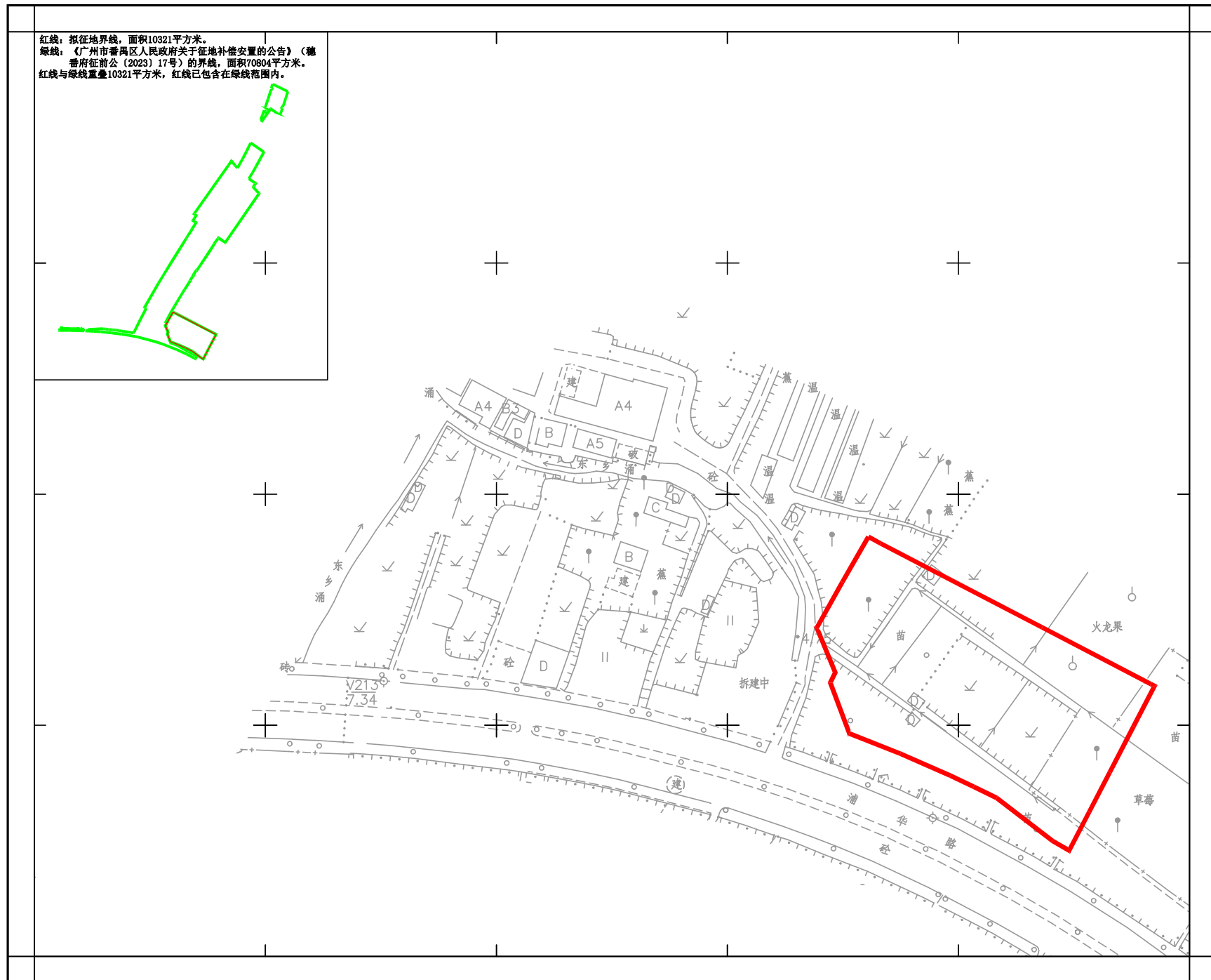
沿线设施用地（海珠湾隧道管理中心）拟征地红线图
